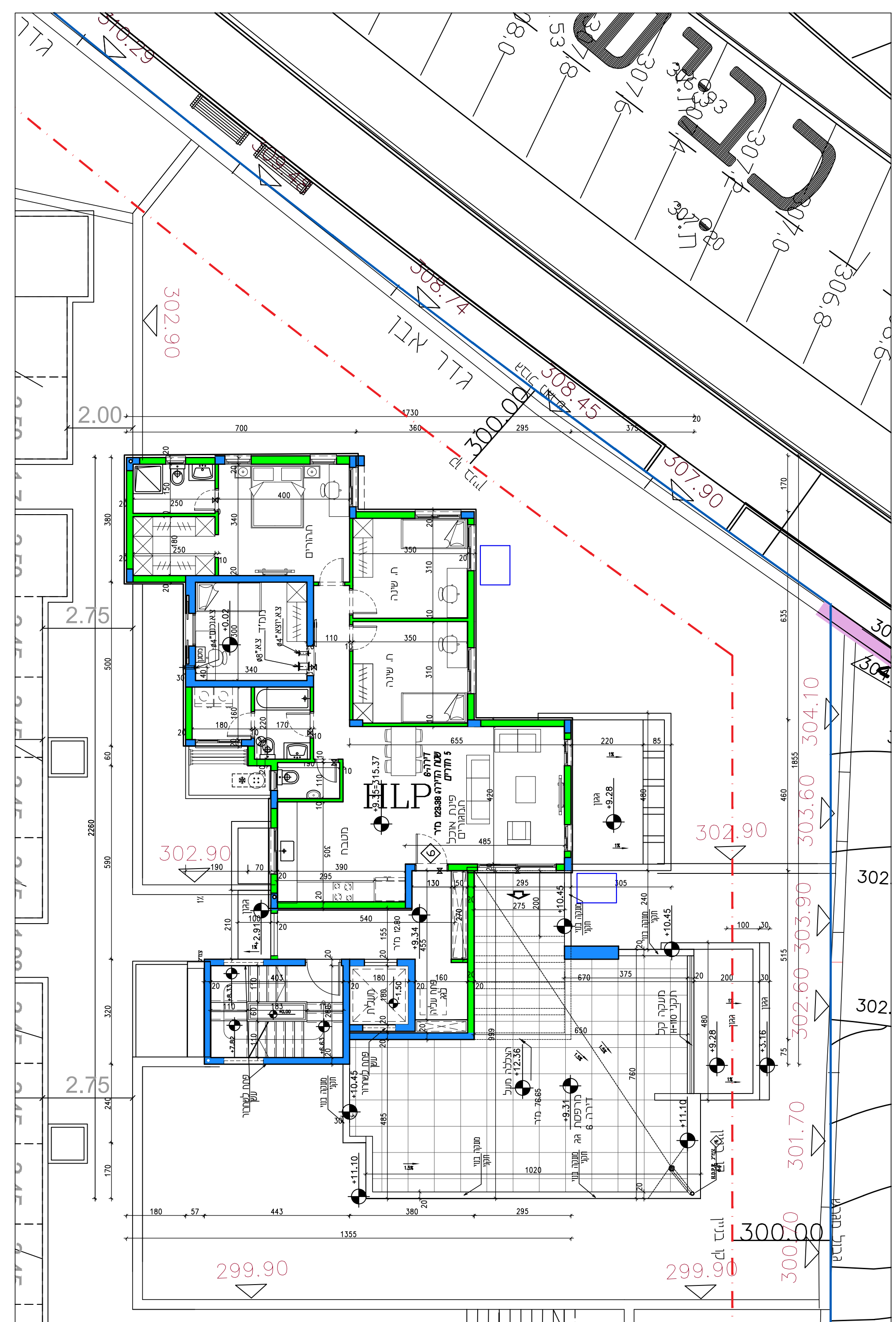
טיפוס 3 P-n תכנית קומה ג' קני"מ 1:100
