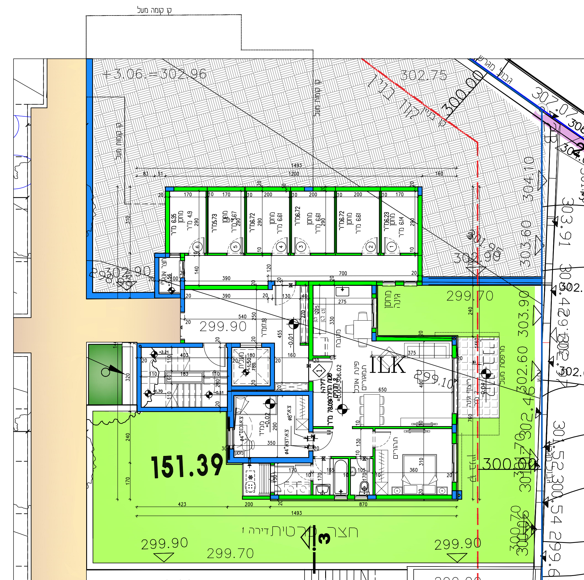
טיפוס 3 P-n תכנית קומת כניסה קני"מ 1:100
