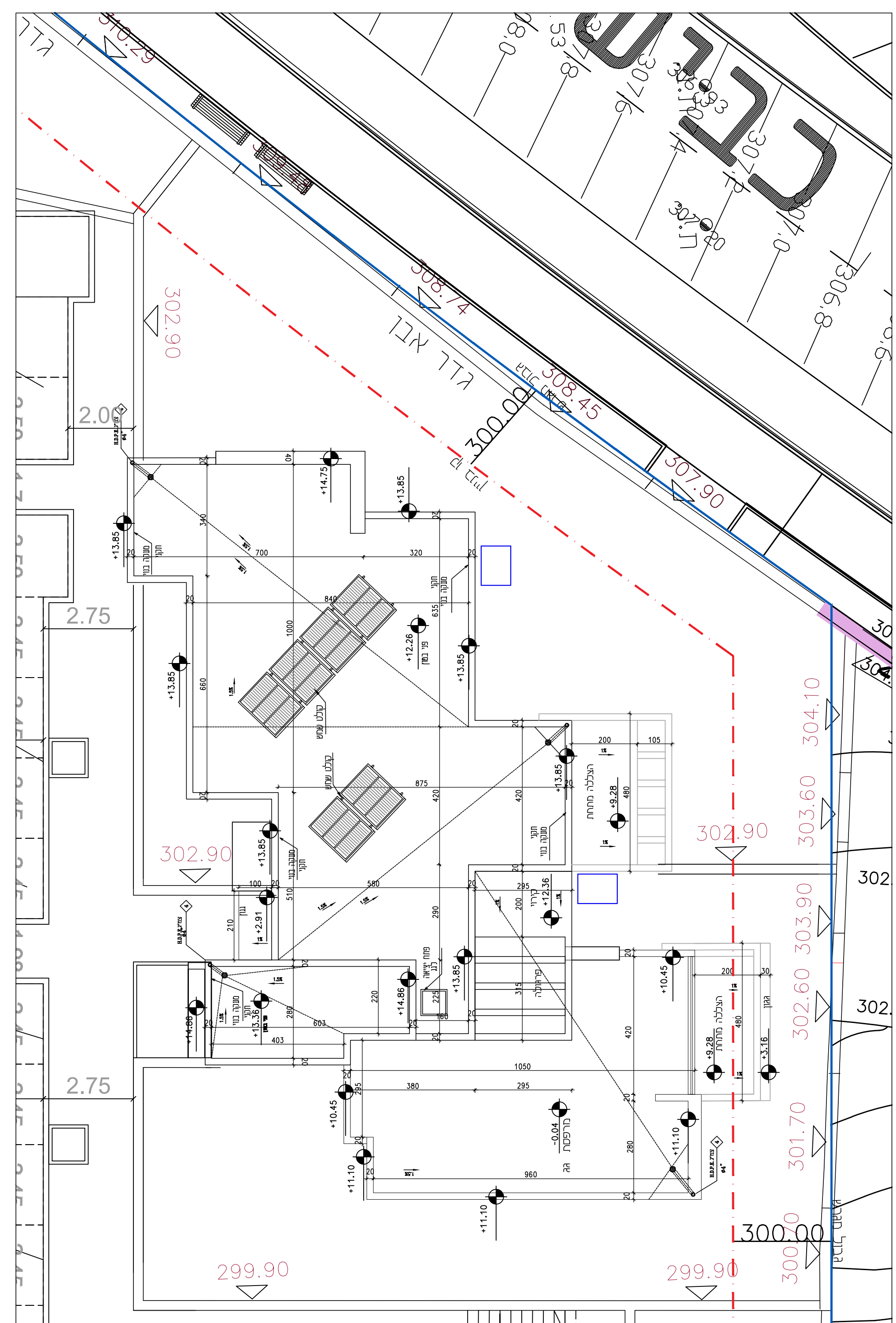
טיפוס 3 P-n תכנית גגות קני"מ 1:100
